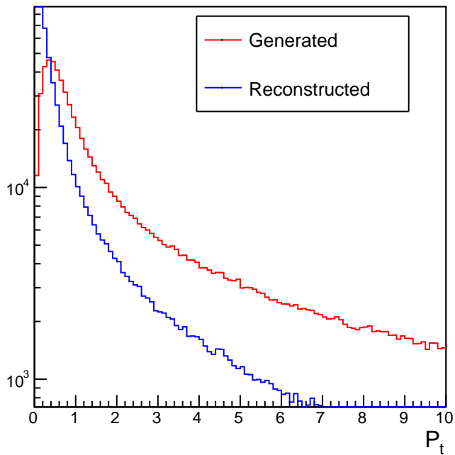
pt_pion_gen
