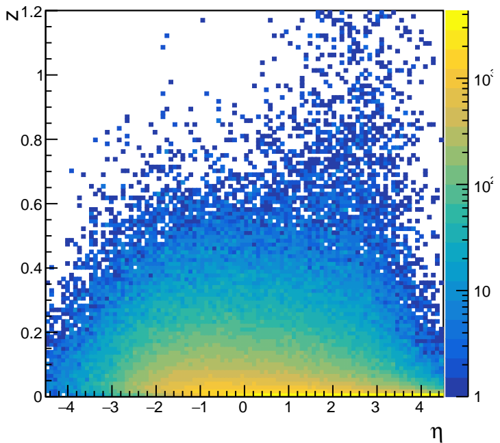
rpion_eta_z
