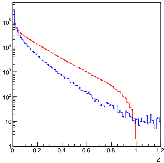
z_pion_gen
