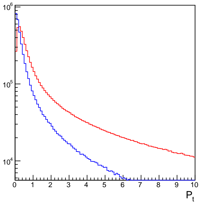
pt_pion_gen
