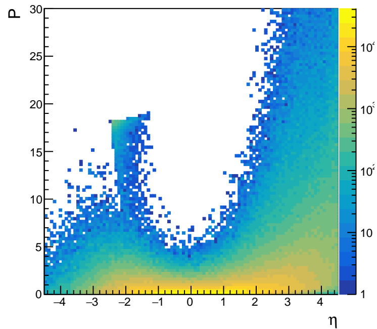
rpion_eta_mom
