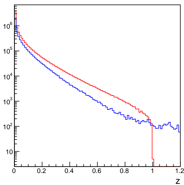
z_pion_gen
